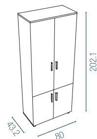
4 melamine doors
