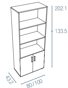
2 melamine doors
