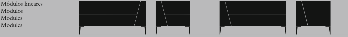
1 Braço à esquerda 1 Brazo a la izquierda Left arm module 1 accoudoir à gauche 1 Braço à direita 1 Brazo a la derecha Right arm module 1 accoudoir à droite H 713 L 1365 P 703 H 713 L 1365 P 703
